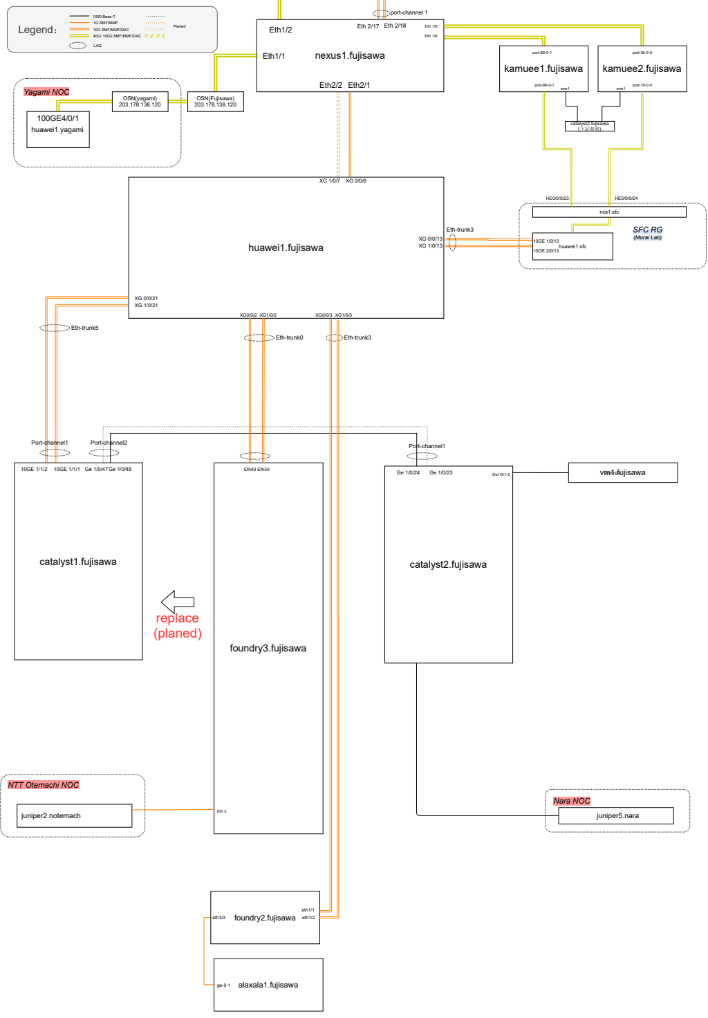
図 10: 藤沢 NOC Layer-1 トポロジ図
