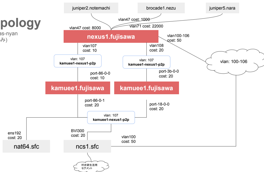
図 11: 藤沢 NOC Layer-3 トポロジ図
