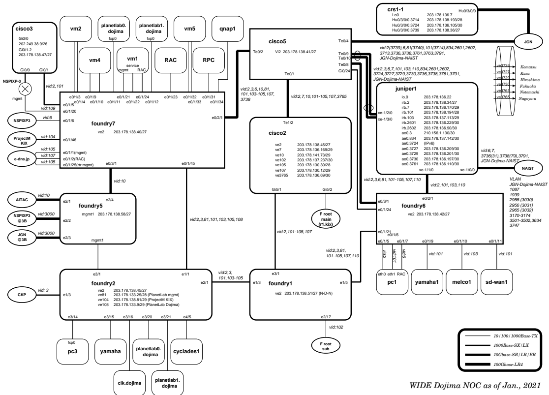
図 13: 堂島 NOC トポロジ
