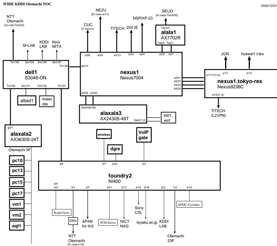
図 6: KDDI 大手町 NOC
