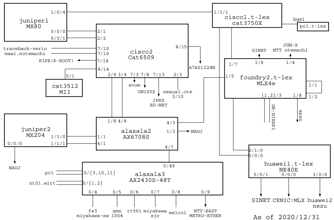
図 5: NTT 大手町 NOC
