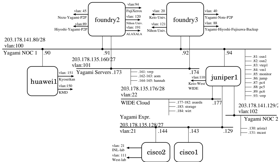
図 9: 矢上 NOC Layer-3 トポロジ
