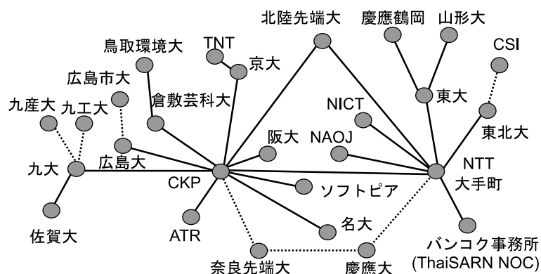
図 3.1. JGN2plus ネットワーク上でのJB プロジェクト構成
