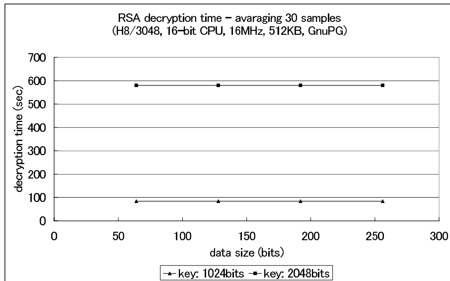
図 2.2. H8/3048 の RSA 復号化の実行時間
