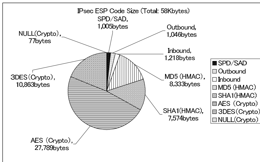
図 2.7. IPsec コードサイズの内訳
