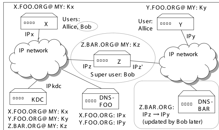
図 5.4. 想定するネットワーク構成
