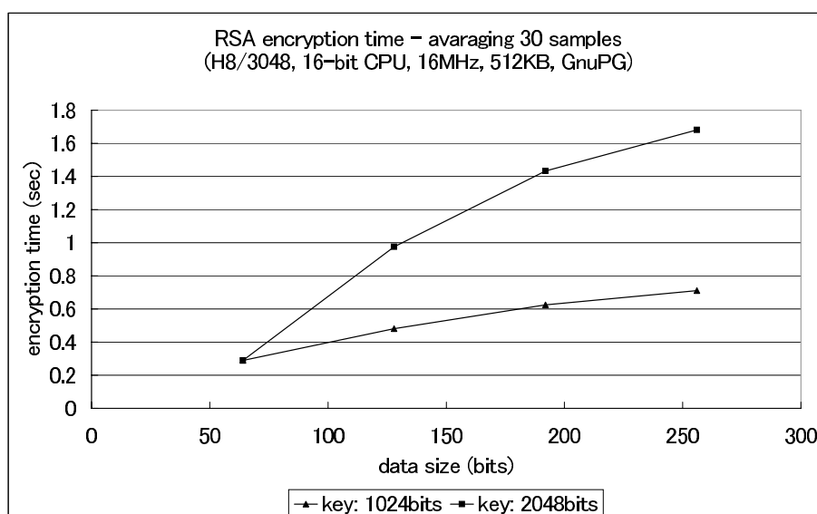
図 2.1. H8/3048 の RSA 暗号化の実行時間
