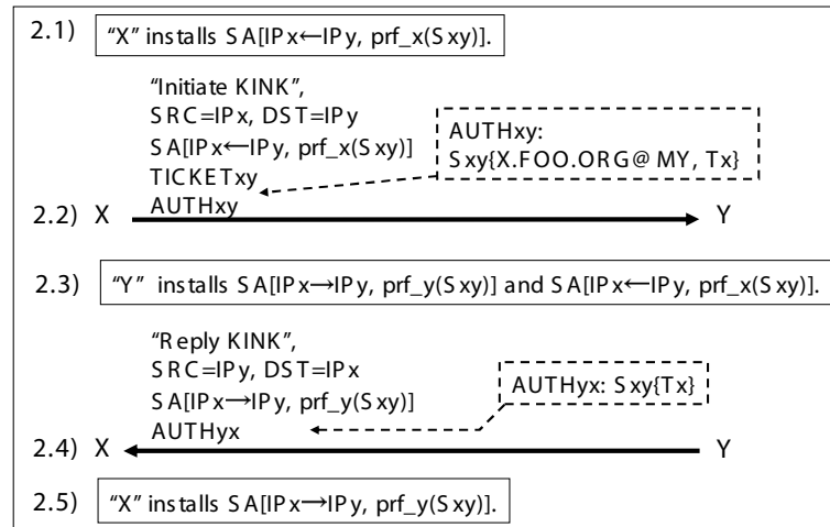
図 5.3. KINK の交換
