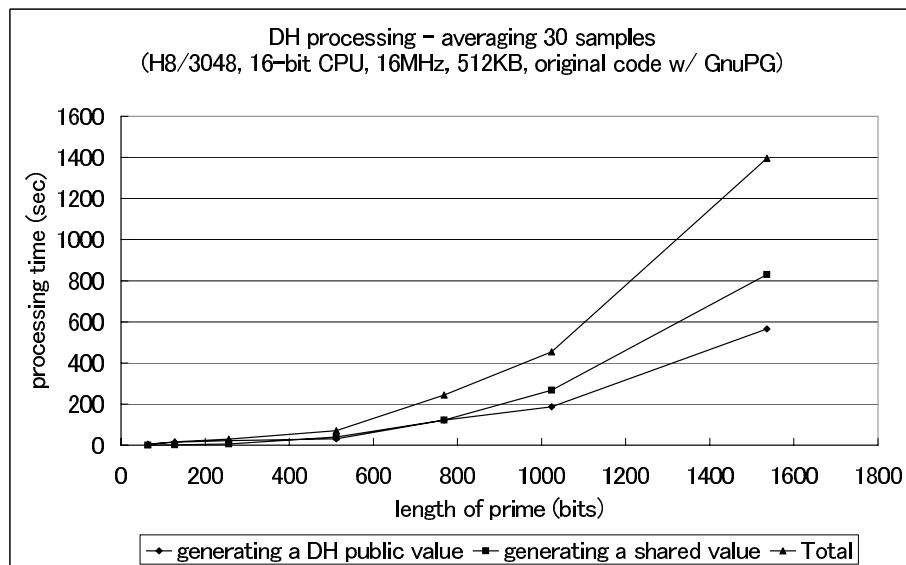
図 2.3. H8/3048 の DH 演算の実行時間
