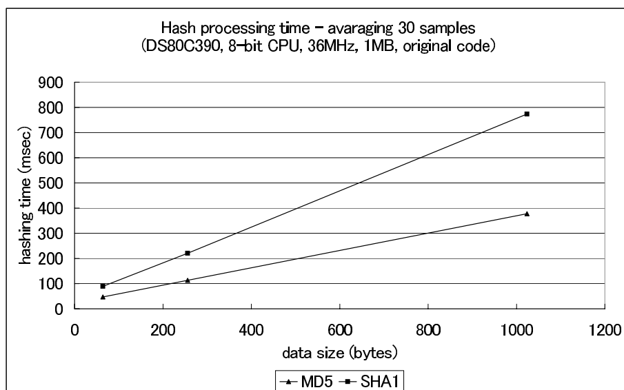
図 2.5. DS80C390 のハッシュの処理時間
