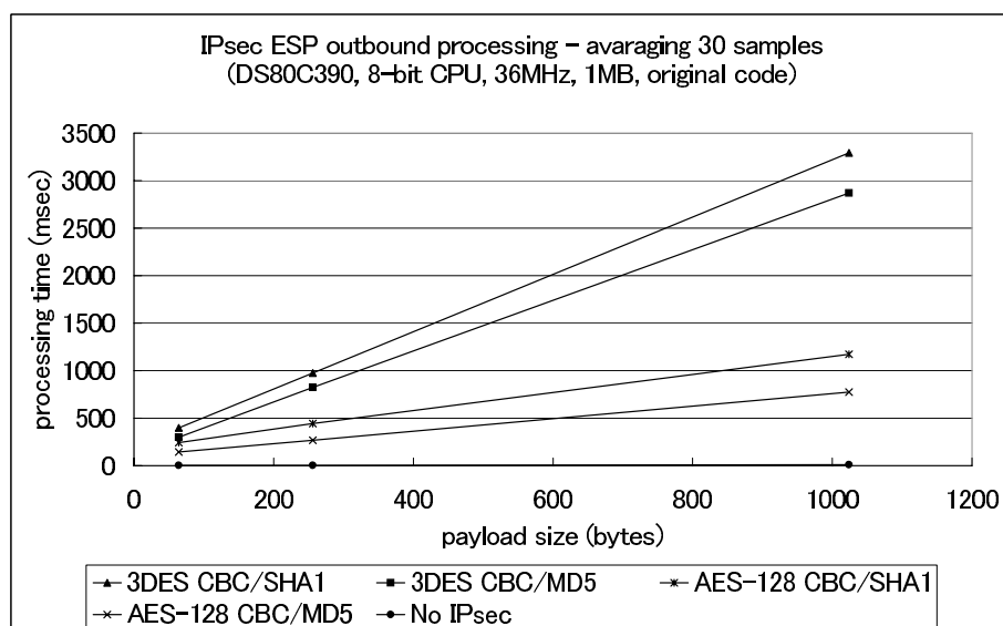
図 2.6. IPsec ESP Outbound 処理の実行時間
