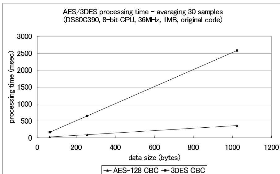
図 2.4. DS80C390 の暗号の処理時間
