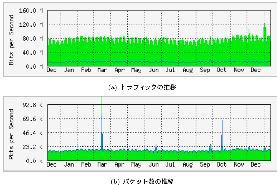
図 2: 2012 年における M-Root DNS 全体の問い合わせ数の推移
