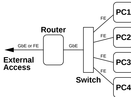
図 1: クラスタ基本構成
