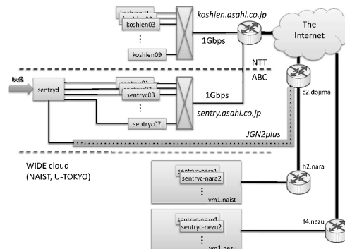
図 3.2. 2010 年度甲子園システムネットワーク概要図
