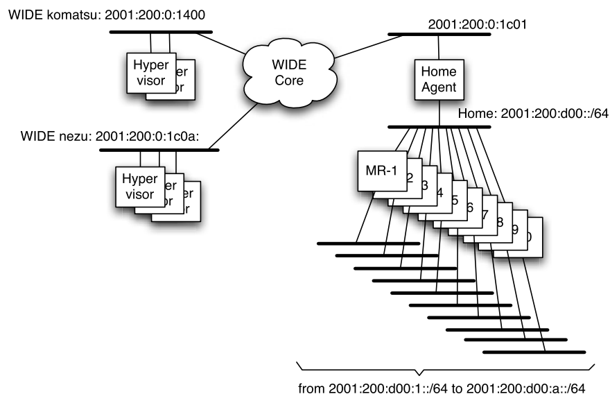
図 6.1. NEMO ベースのネットワーク可搬性を実現した WIDE Cloud のトポロジ
