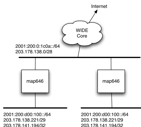
図 7.1. WIDE Cloud における NAT64 サービスのトポロジ
