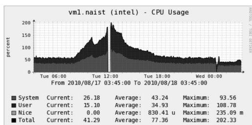
図 3.6. VM 応答悪化時の Hypervisor の CPU 使用率
