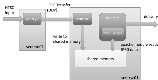
図 3.1. sentry サーバプログラムの動作
