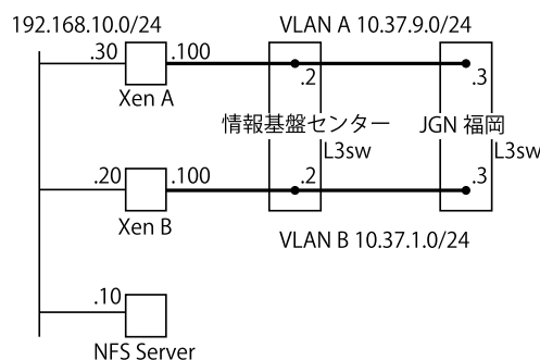
図 4.2. Xen におけるライブマイグレーション実験時のネットワーク構成
