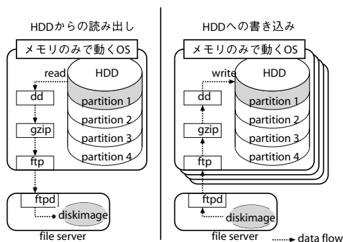
図 3.2. ハードディスクへの OS 導入
