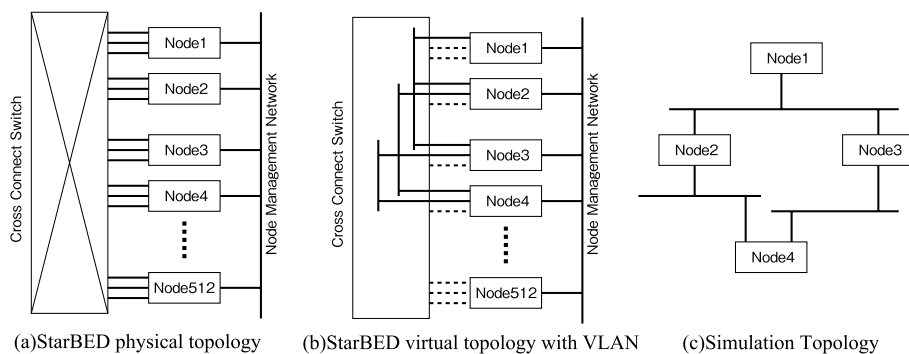
図 2.1. StarBED の概念的トポロジとシミュレーション環境への適応
