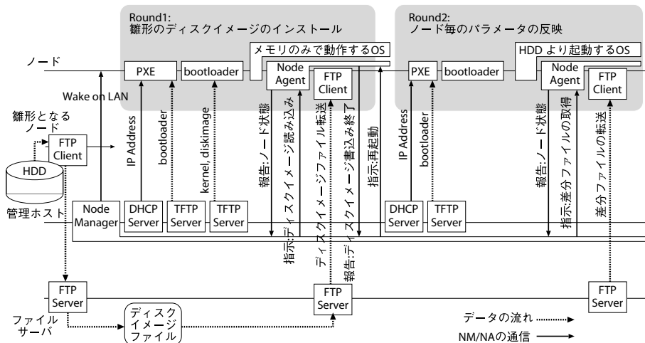
図 3.3. ハードディスクを用いる OS の動作するノードへの OS 配布
