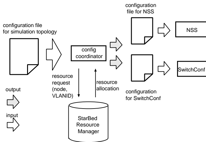
図 3.1. シミュレーション環境構築までの流れ
