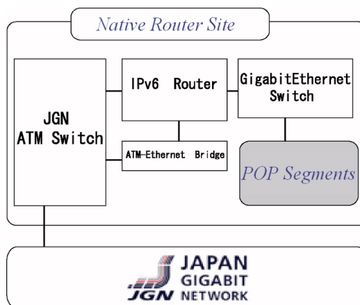
Fig. 3.4. Default configuration of router site
